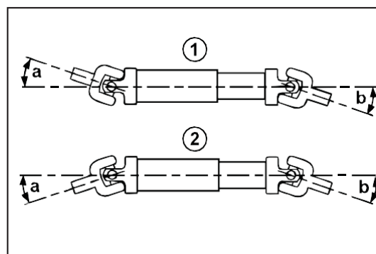
Slika 2.39 (d) Zglobna veza na teleskopskom pogonu pravilno poravnatim viljuškama 1 - izgled Z oblika 2 - izgled W oblika
